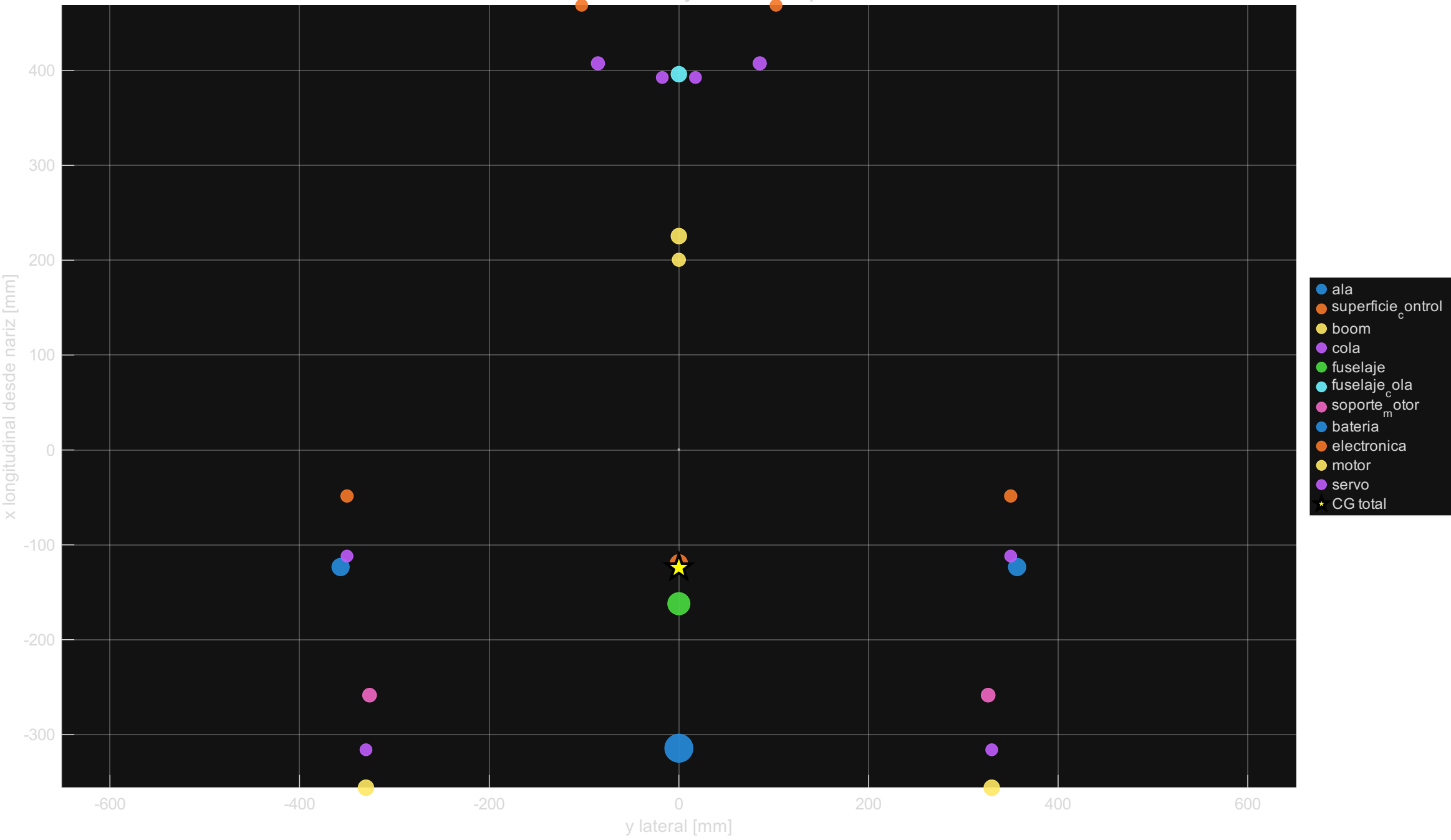
Distribucion de masa y CG -vista superior
